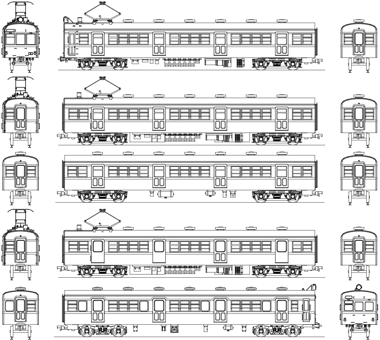
上記図面は 国鉄 73 系「片町線タイプ」5 輛セット の内容です
