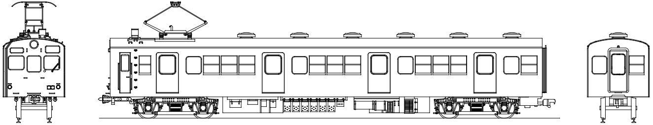
図面はクモハ 73-近代化改造車・大鉄通風器付きです
